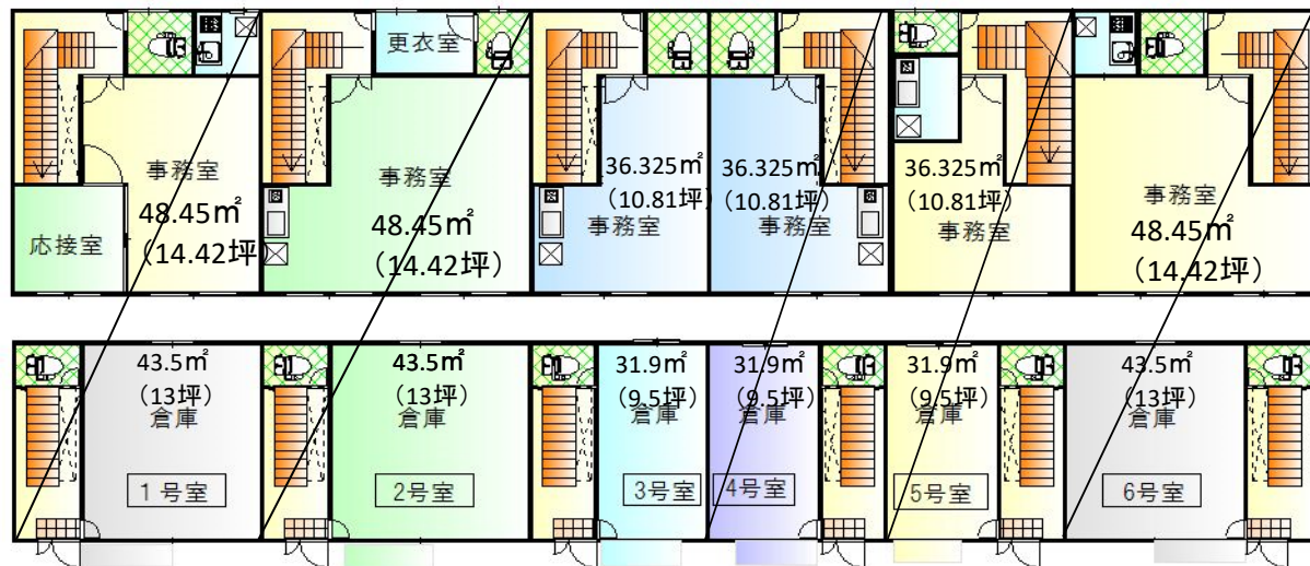
▲間取り図
