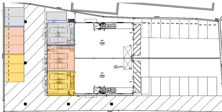
配置図
