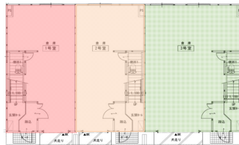
1F平面図
