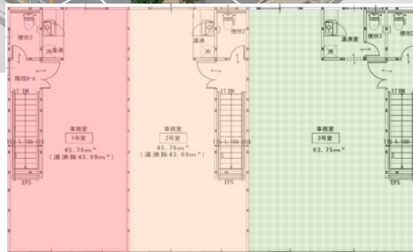
2F平面図
